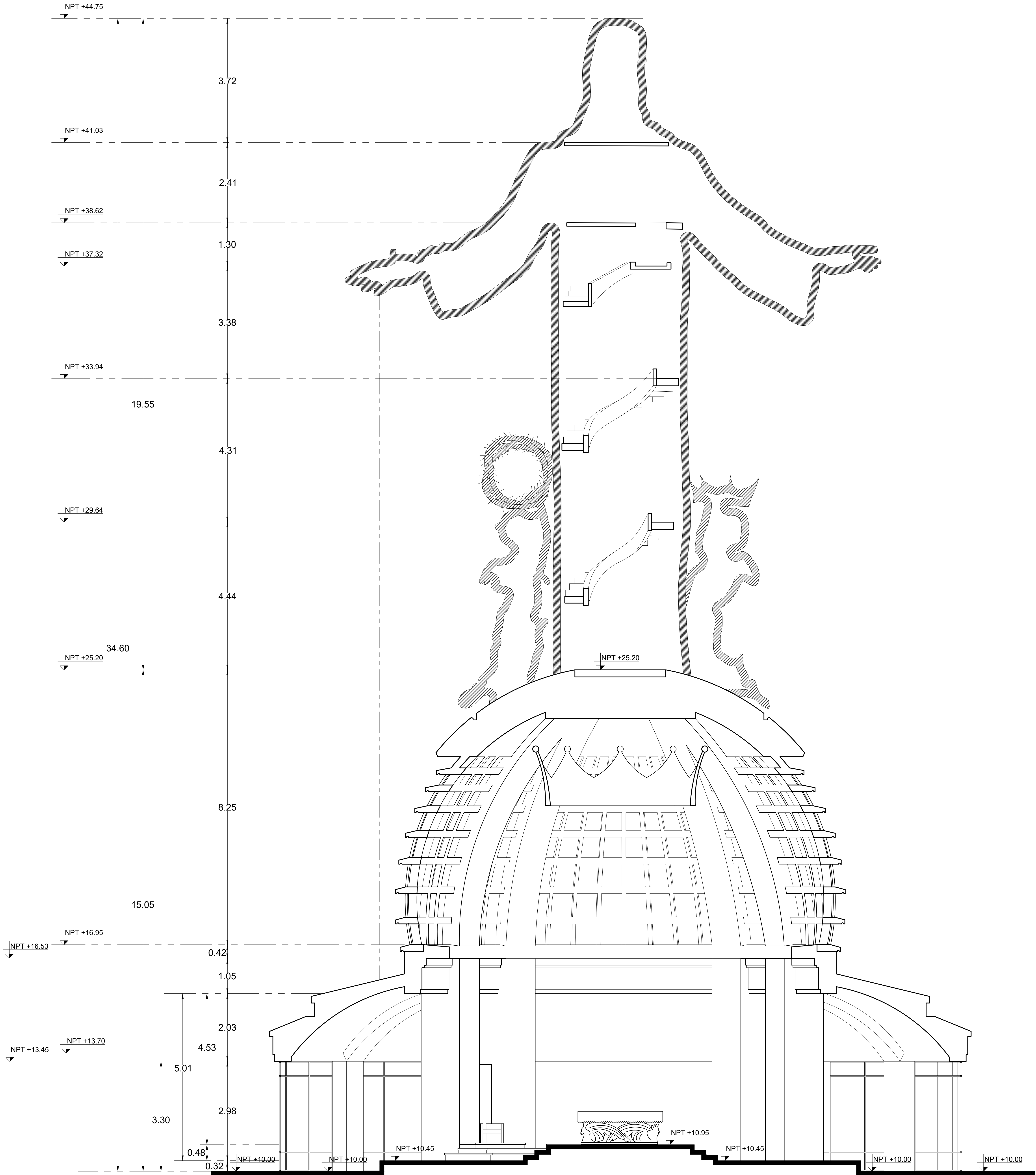
CORTE 02 ESCALA 1:50
